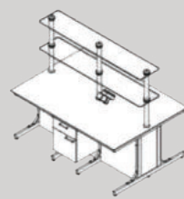
L01-42 Masă pentru elevi (fizică) Dimensiuni: 182x130x75/157 (LxIxH)
