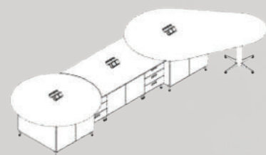
L01-12 Masă pentru elevi (fizică) Dimensiuni: 488x196x75 (LxIxH)
