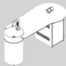
L01-73 Masă pentru profesor Dimensiuni: 154x80x75 (LxlxH)
