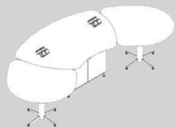
L01-22 Masă pentru elevi (fizică) Dimensiuni: 359x174x75 (LxlxH)
