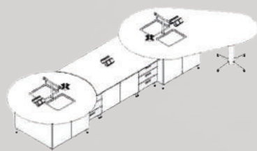
L01-11 Masă pentru elevi (chimie-biologie) Dimensiuni: 488x196x75 (LxlxH)
